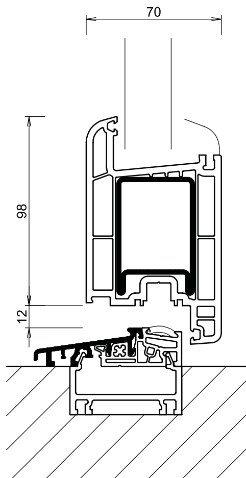
Hoja de Puerta F90-13-0116 Umbral F00-84-9880
