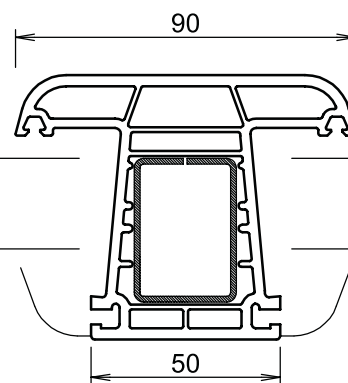
Poste F90-15-0122
