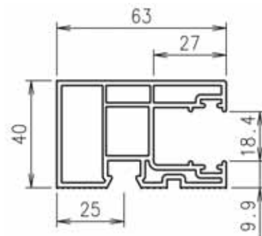
4131 Guía 14 mm
