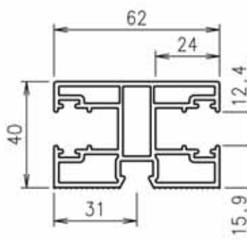
4132 Guía doble 8 mm
