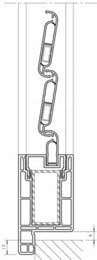
Sección vertical. Lamas móviles
