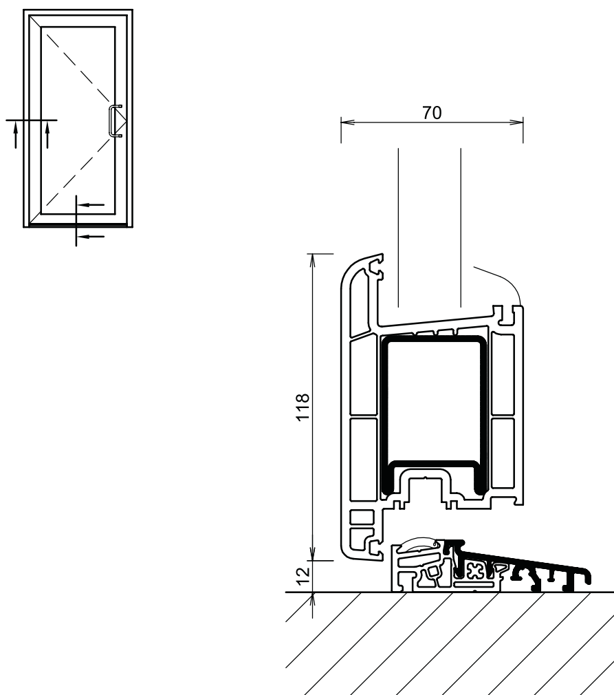
Hoja de Puerta F90-13-0115 Umbral F00-84-9880
