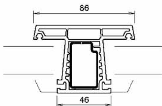
Poste F40-15-1422.W
