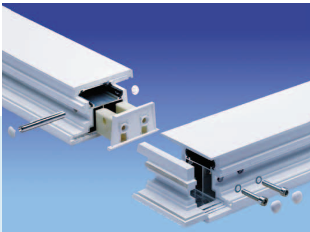
Detalle de unión de las esquinas
